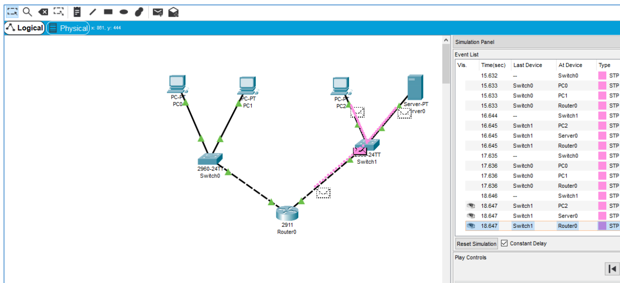
Рисунок 3 – Работа симуляции Cisco Packet Tracer
